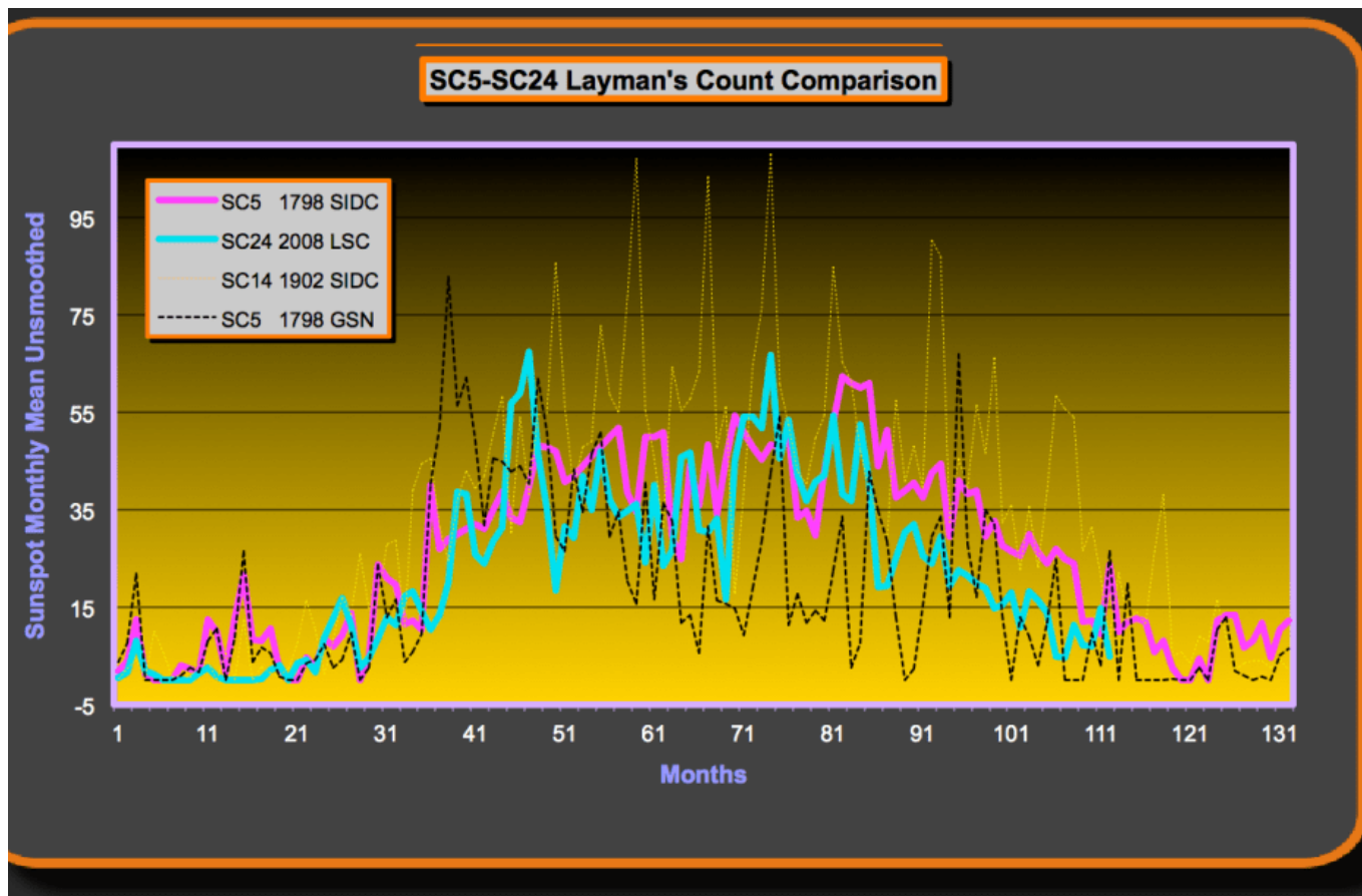
Confronto tra i due cicli, il ciclo 5 (minimo di Dalton linea di colore fucsia) e il ciclo 24 (ciclo attuale linea di colore azzurro) per il metodo di conteggio del Layman's Sunspot Count
