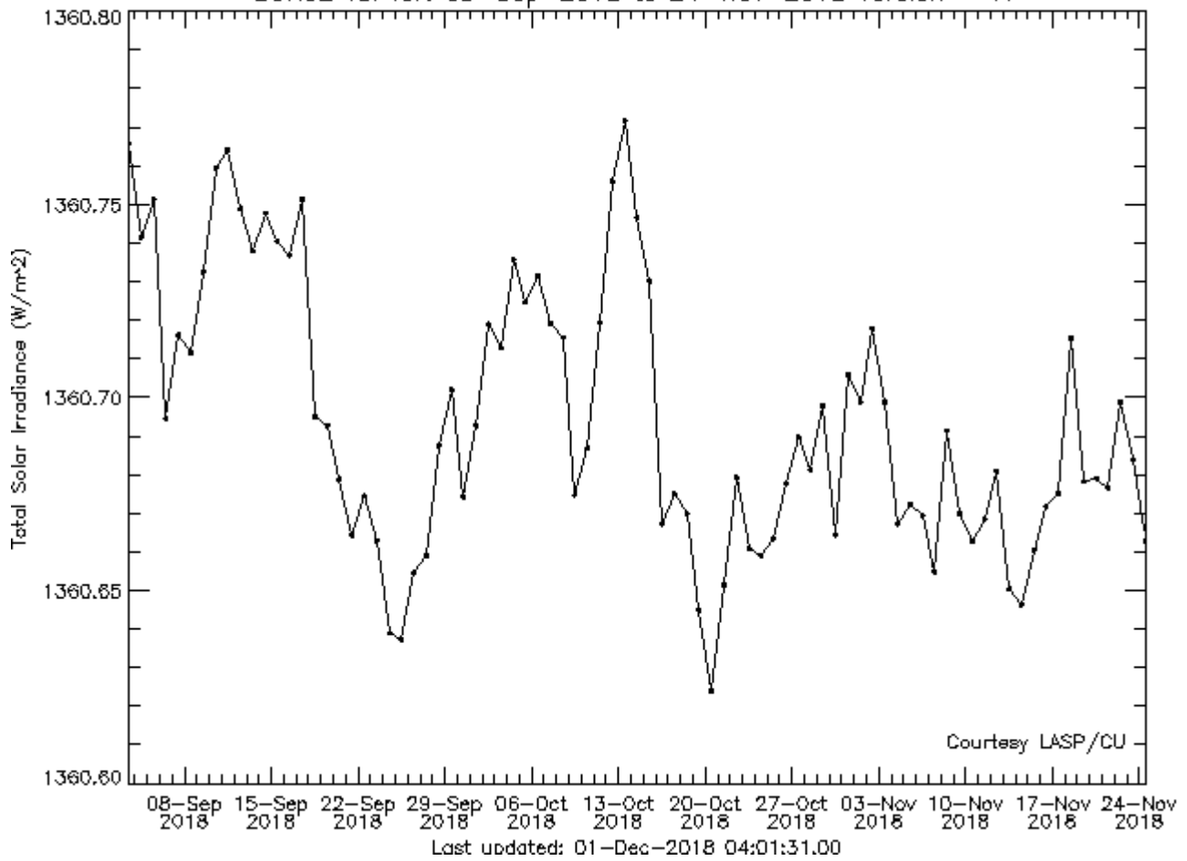
Grafico della Total Solar Irradiance (TSI)
